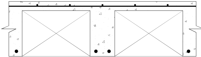
Figura 9.2. Solaio misto.
