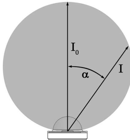
Figura 1.3. La ripartizione “lambertiana” di un LED ( I = I_0 \cos \alpha )
