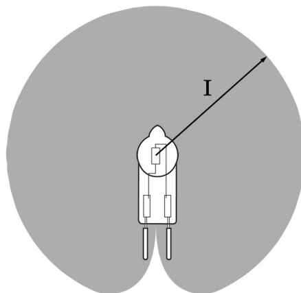
Figura 1.2. Ripartizione nello spazio del flusso luminoso emesso da una sorgente ad alogeni da 12 V con bulbo rivestito di cerio
