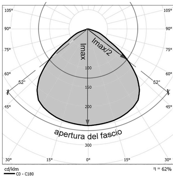
Figura 1.6. Diagramma polare del solido fotometrico di un apparecchio avente per sorgente un LED dotato di una lente con la quale l'apertura del fascio è 104^\circ
